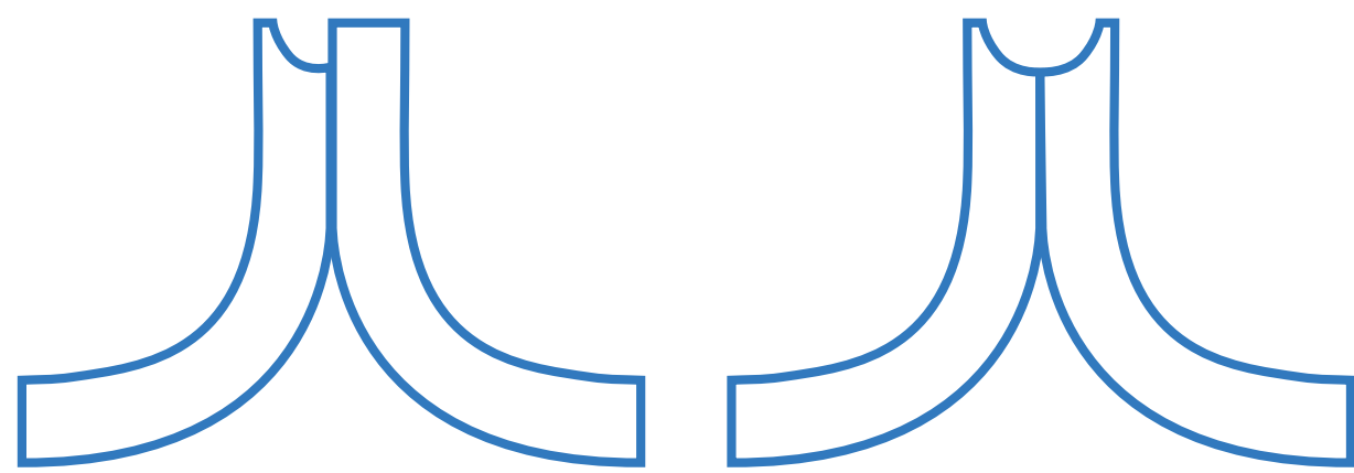
J Groove
